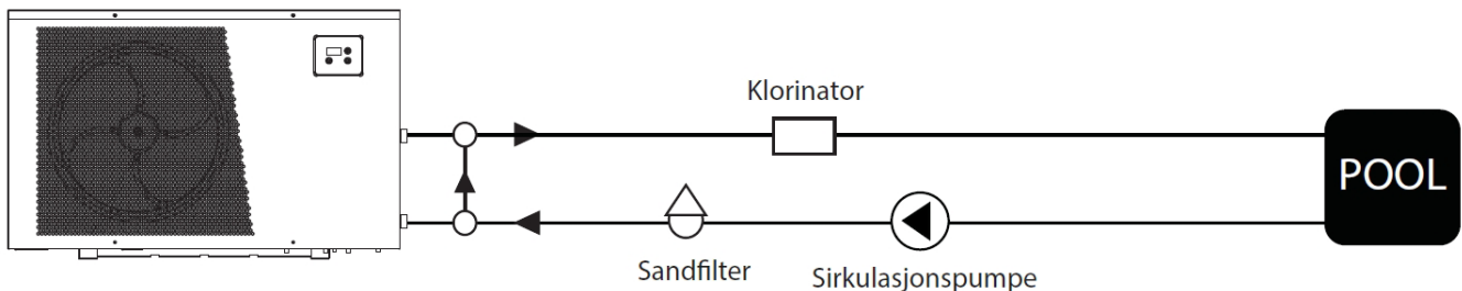
Prinsipskisse for installasjon
